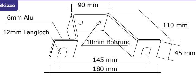
Wandhalter Skizze
