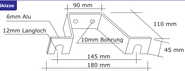
Wandhalter Skizze
