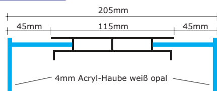
Profil Skizze
